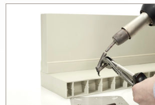
CORRECTA INSTALACIÓN SOLDADURA-CABEZAL
