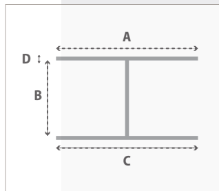
Paneltim® PP Н профиль
