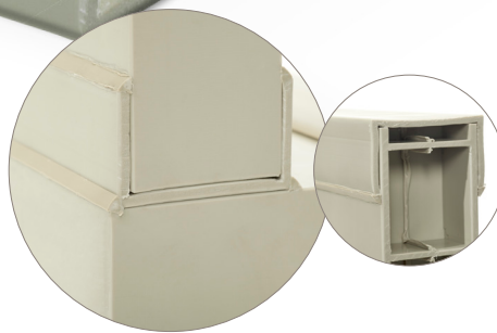
PP U ПРОФИЛЬ для соединения панелей и закрытия открытых ячеек
